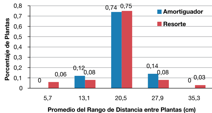
Figura 3. Porcentaje de semilla en función de la distancia entre plantas (cm) con copiado a través de resorte tradicional y de amortiguador con carga constante.
