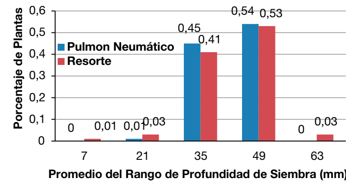
Figura 5. Porcentaje de semillas contabilizadas en función de la profundidad (mm) y del sistema de copiado a través de resorte tradicional y de Pulmón Neumático, regulada para lograr 5 cm de profundidad.
